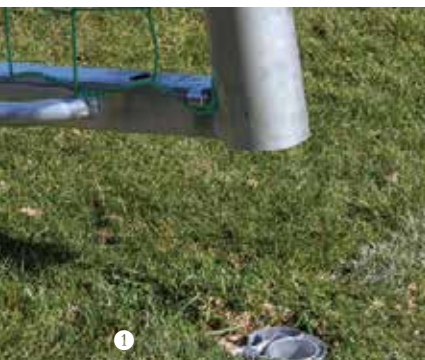
Per Knopfdruck kann der Adapter ausgefahren werden.
