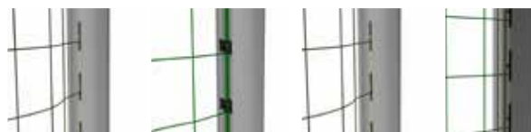
Eingefräste Netzaufhängung Kunststoff-netzhaken Alu Entnahmesicherung FLEX Entnahmesicherung
