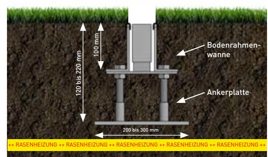
Revisionsschacht im Bodenrahmen
