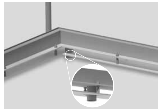
Revisionsschacht im Bodenrahmen
