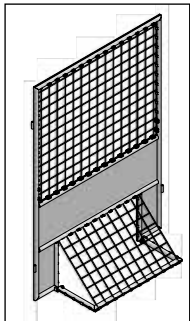
Torelement (2x)
