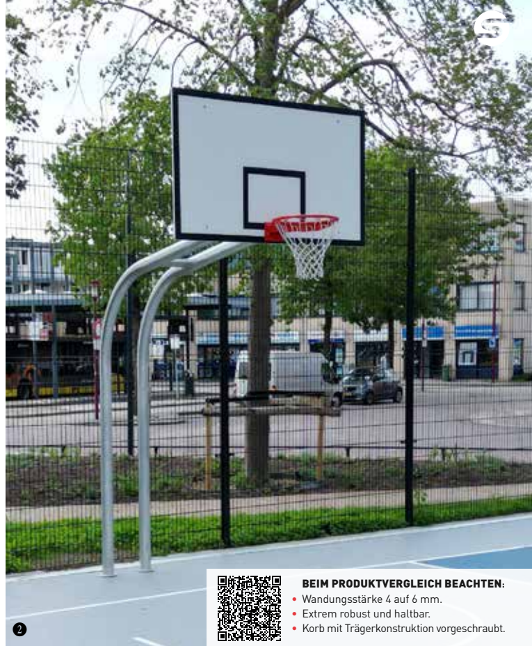
Typ B, Multiplex-Zielbrett mit Gummikante, Korb pulverbeschichtet mit Nylonnetz.
