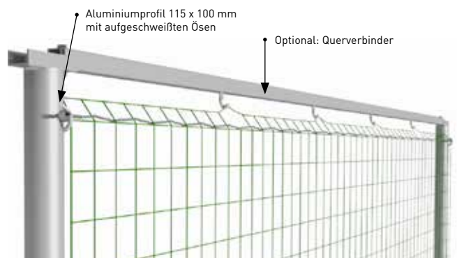
Ballfangzaun „Standard“ mit Querverbinder und Schrägstütze.
